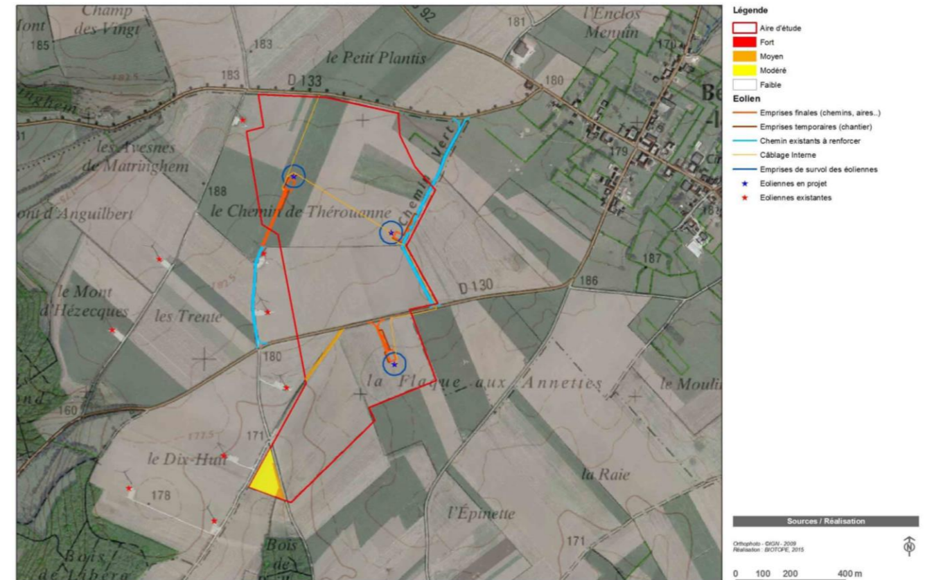
Carte 10 : Sensibilité prévisible de l'avifaune et confrontation avec le projet (source : Biotope, 2016)
