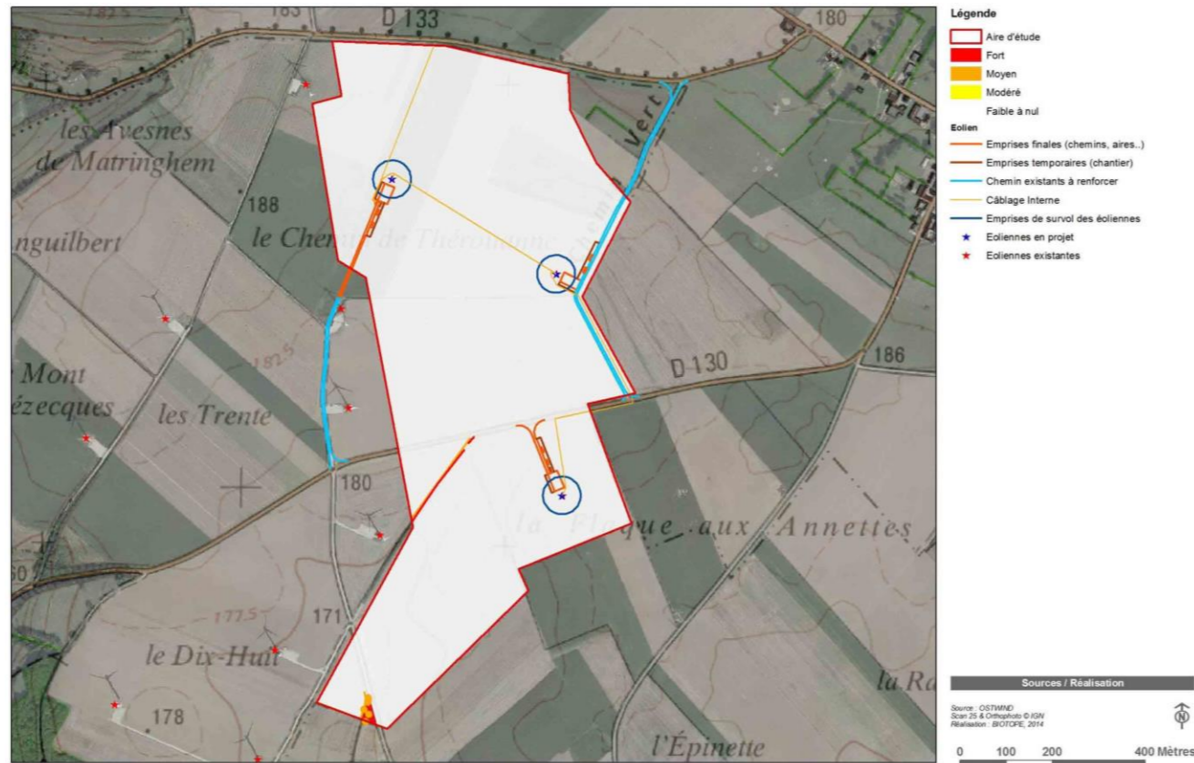
Carte 9 : Sensibilité prévisible de la flore et confrontation avec le projet (source : Biotope, 2016)
